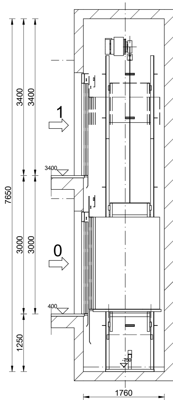
ΤΟΜΗ ΦΡΕΑΤΟΣ : 1:50
