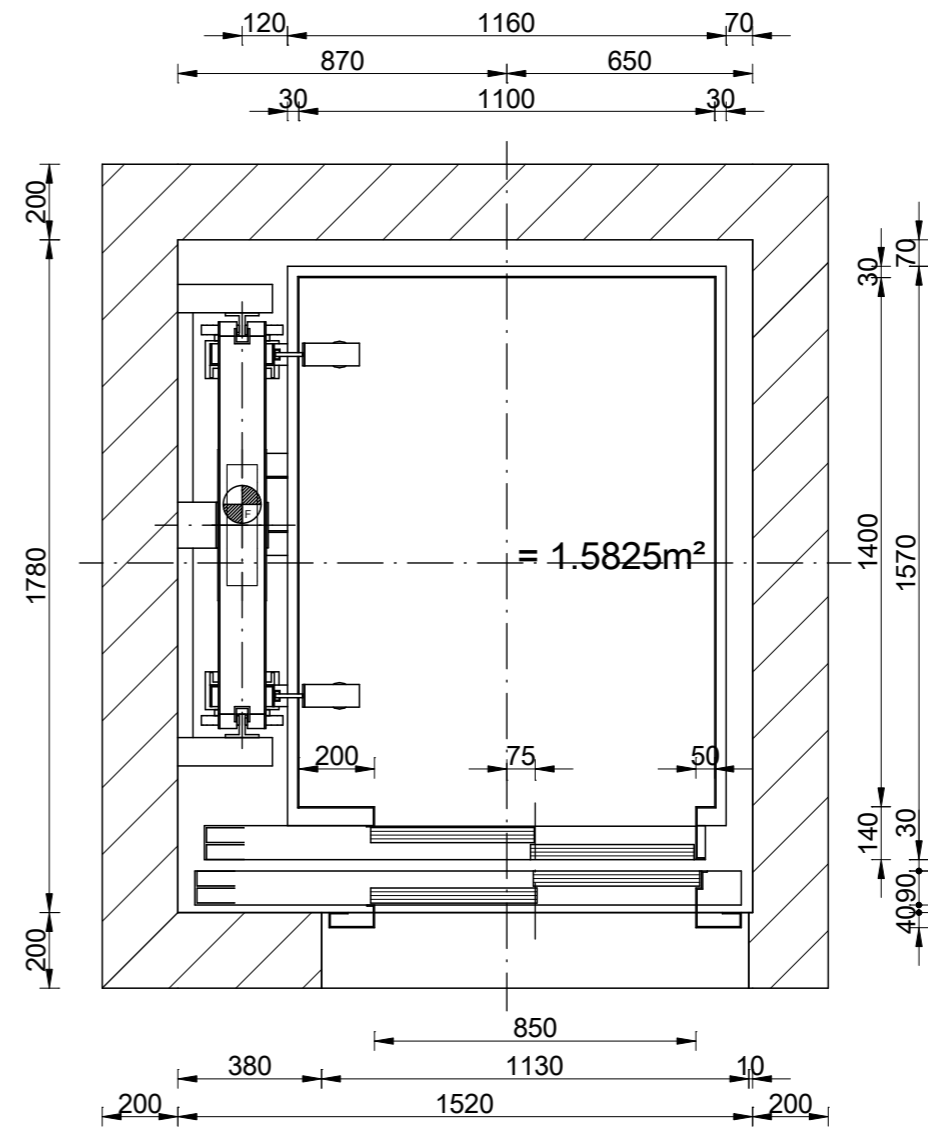
: 1:20 ΚΑΤΟΨΗ ΦΡΕΑΤΟΣ
