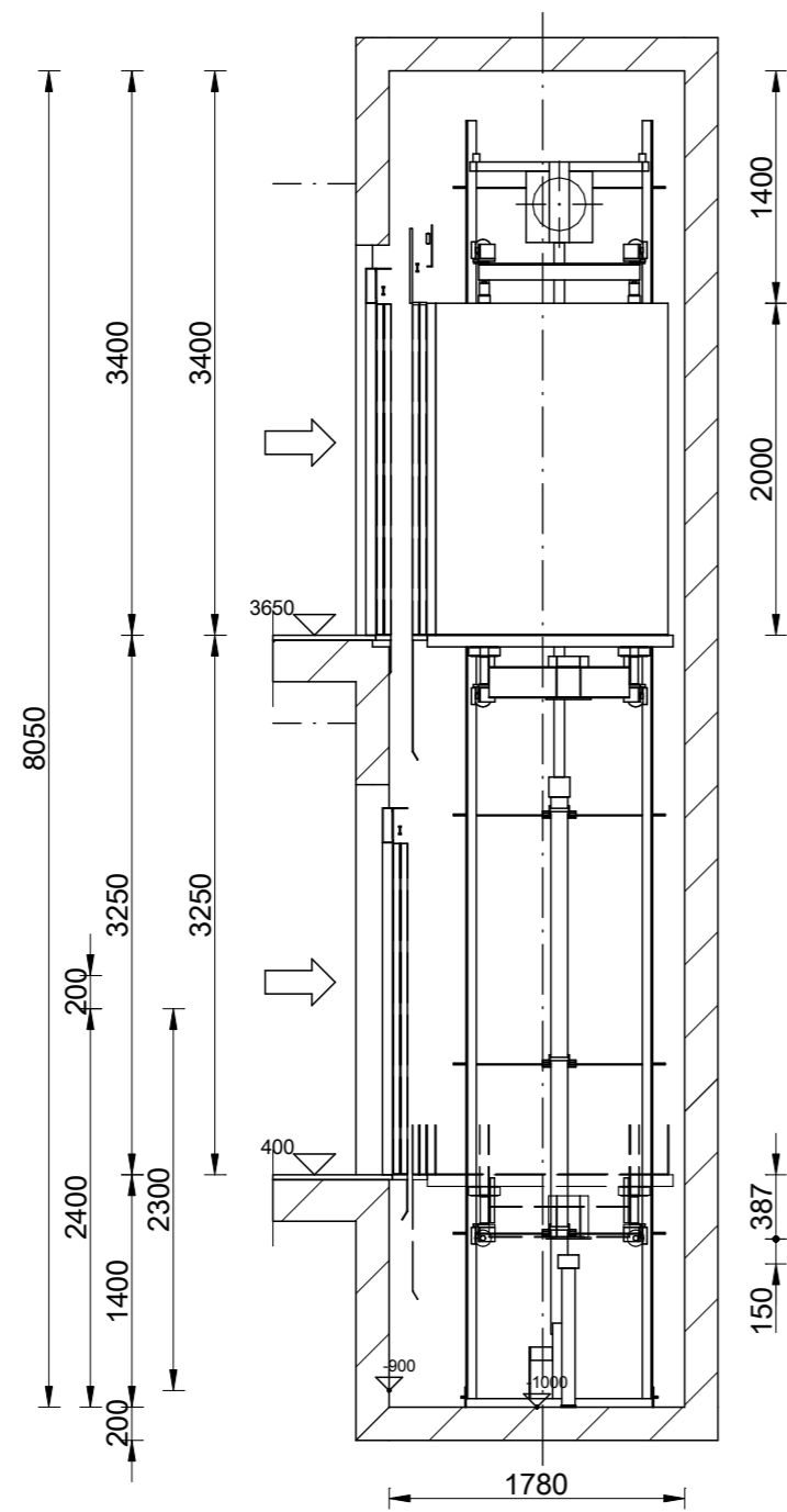
ΤΟΜΗ ΦΡΕΑΤΟΣ : 1:50
