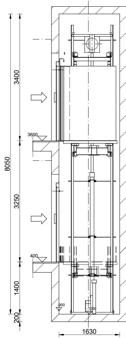
ΤΟΜΗ ΦΡΕΑΤΟΣ : 1:50
