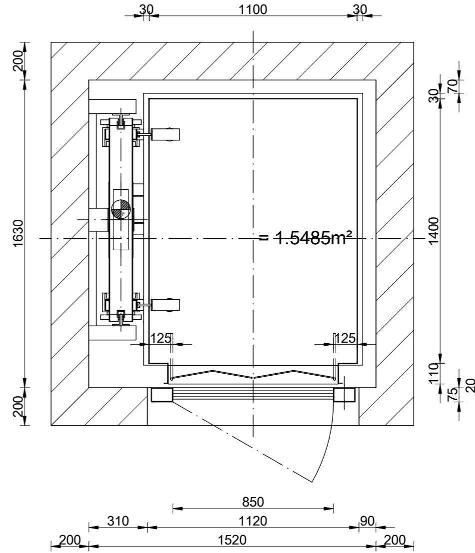
: 1:20 ΚΑΤΟΨΗ ΦΡΕΑΤΟΣ
